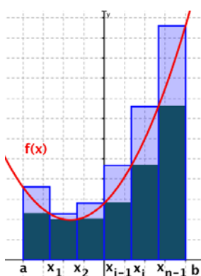
Suma inferior y superior con la partición P_1
